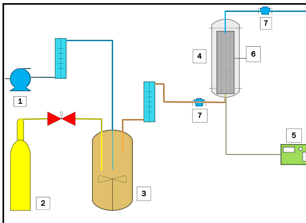
شکل ۱. پابلوت نمونه برداری (۱): پمپ دمنده هوا ۲: کپسول گاز سولفید هیدروژن ۳: محفظه اختلاط ۴: گرمکن ۵: ترموستات و سیستم کنترل دما ۶: راکتور ۷: پورت های نمونه برداری
