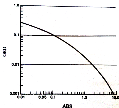
شکل ۱: منحنی تصحیح استغراق برای اسکرابرهای بسترار که به روش تصادفی پر شده‌اند [۱۴]
