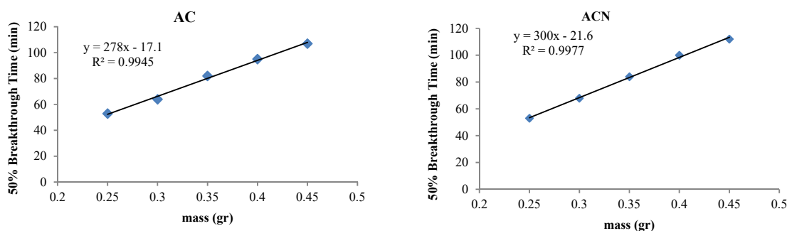
شکل (۷) - نمودار زمان نقطه شکست ۵۰ درصد سووفلوران روی جاذب های AC و ACN در مقابل جرم
